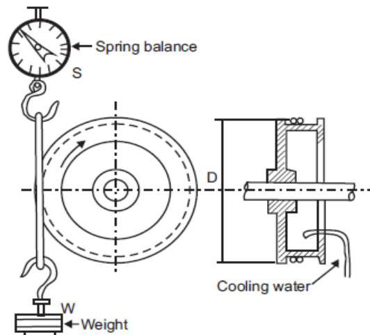
Fig. 30. Rope brake
