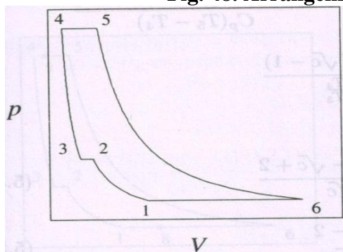
P-V diagram
