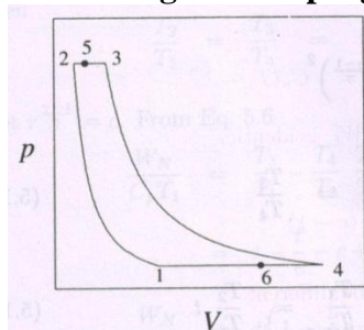
P-V diagram
