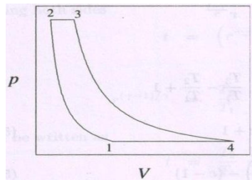
P-V diagram
