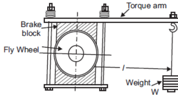
Fig. 29. Prony brake
