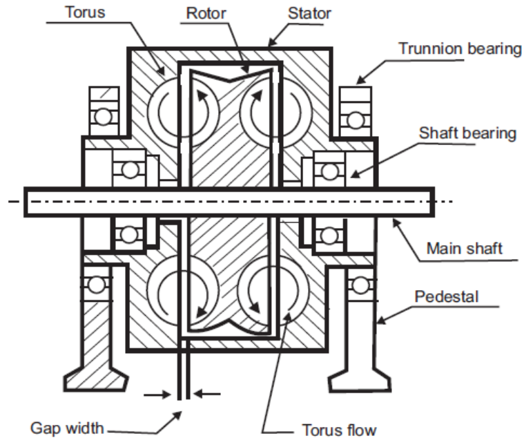
Fig. 31. Hydraulic dynamometer
